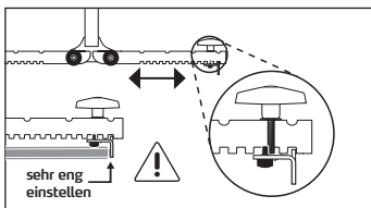
Haltebacken möglichst eng einstellen
