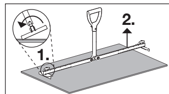
Leichtes Lösen von der Fliese
